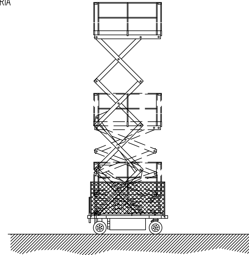
Plataforma elevadora móvil de tijera
