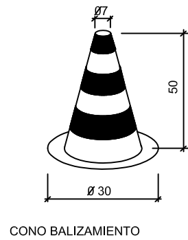
CONO BALIZAMIENTO
