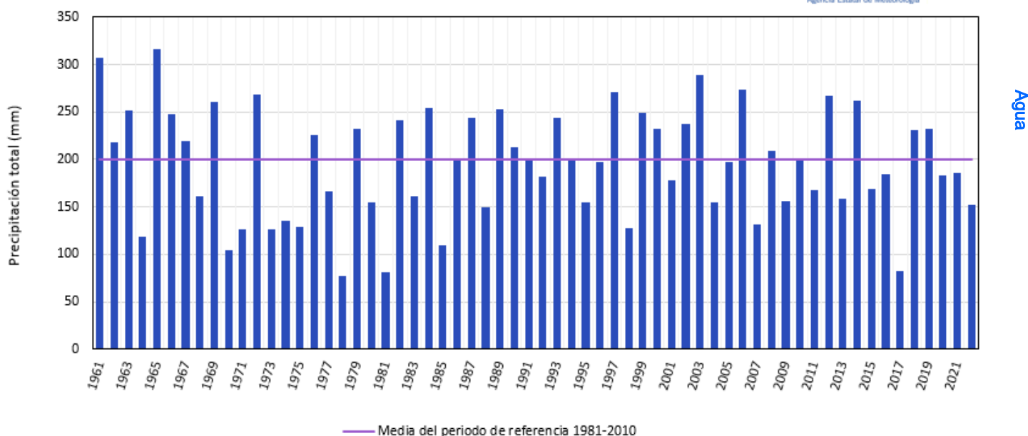
Precipitación OTOÑO España peninsular
