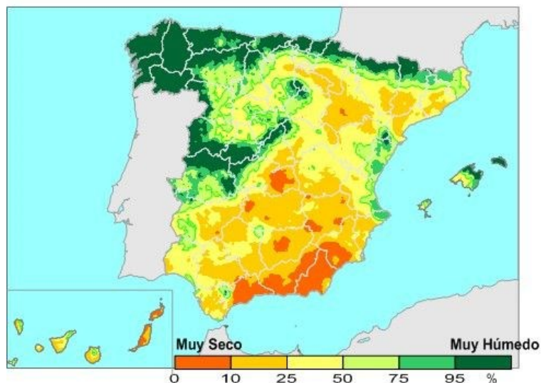
%RESERVA DE HUMEDAD DEL SUELO SOBRE LA CAPACIDAD MÁXIMA A 30/11/2022
