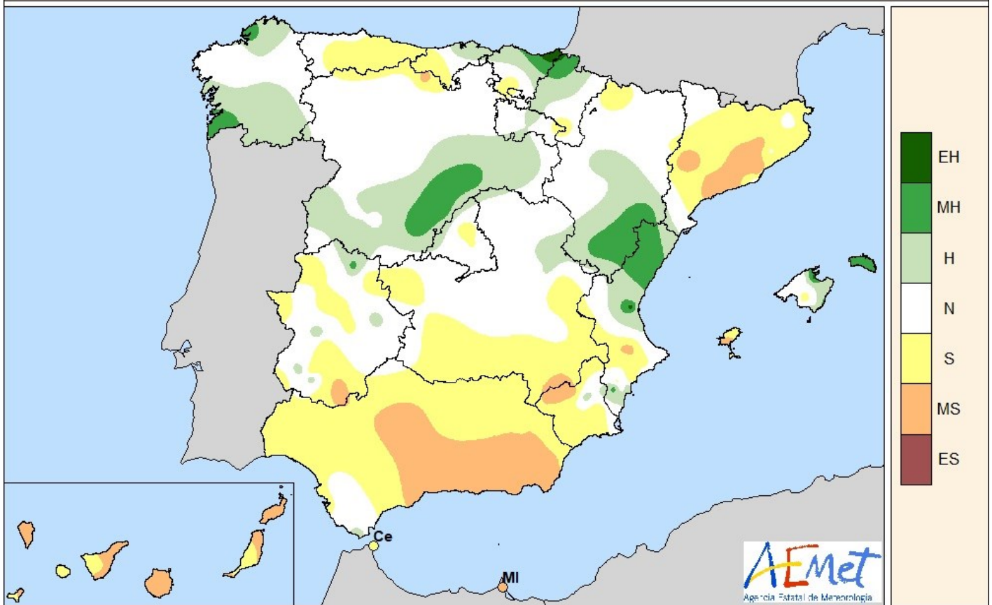
CARÁCTER DE LA PRECIPITACIÓN - NOVIEMBRE 2022
