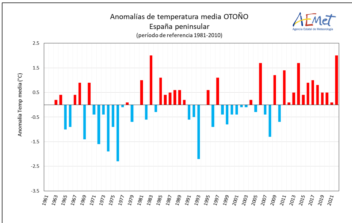
Serie de anomalías de la temperatura media del otoño en la España peninsular desde 1961 (periodo de referencia 1981-2010)
