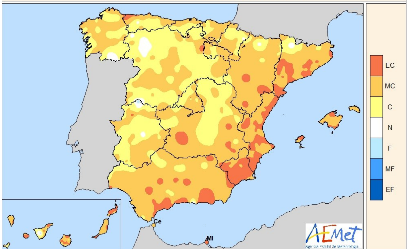
CARÁCTER DE LA TEMPERATURA - NOVIEMBRE 2022
