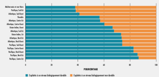
FIGURE 15 PROPORTION DES STOCKS EXPLOITÉS À DES NIVEAUX BIOLOGIQUEMENT DURABLES ET NON DURABLES, PAR ZONE STATISTIQUE DE LA FAO, EN 2015
