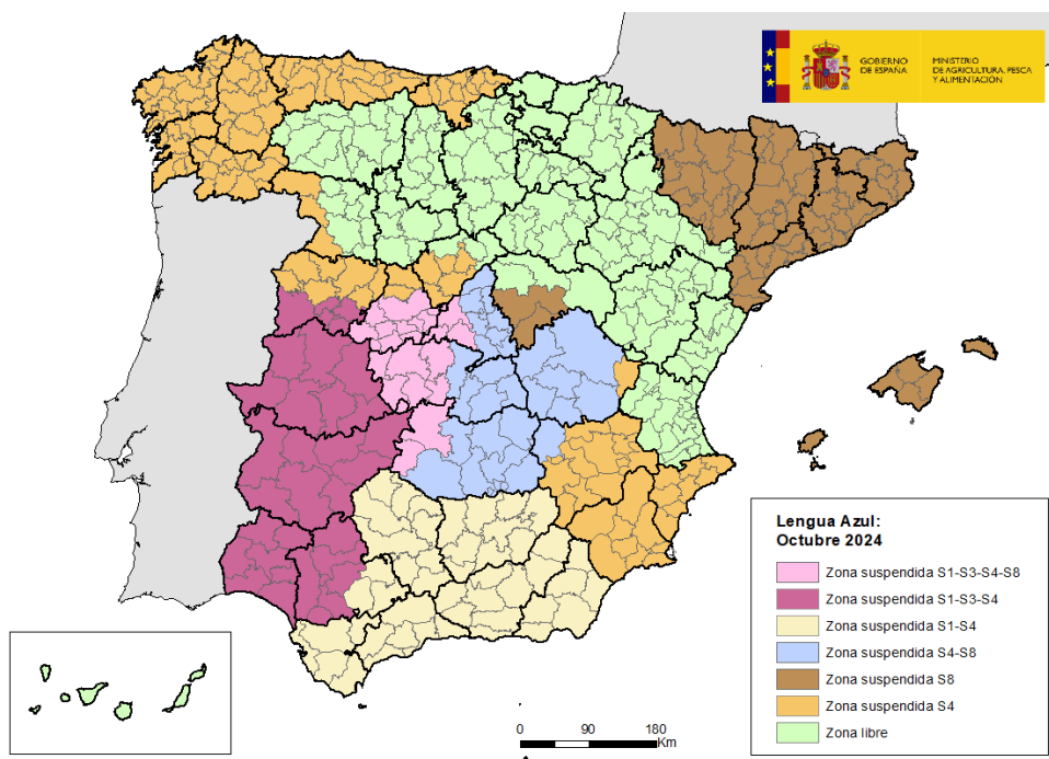
Mapa 2: Zonas suspendida por diferentes serotipos del virus de la lengua azul, octubre 2024.
