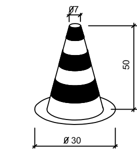
CONO BALIZAMIENTO
