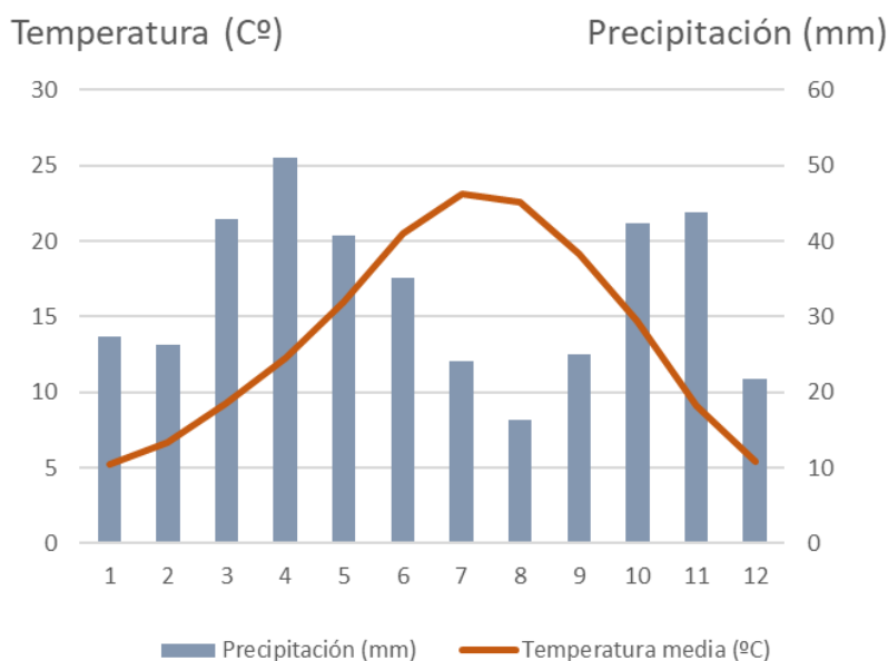
Figura 3.1. Climograma: temperaturas medias mensuales (Cº) y precipitaciones medias mensuales (mm) registradas en la estación de El Bayo en el periodo 2005-2021.
