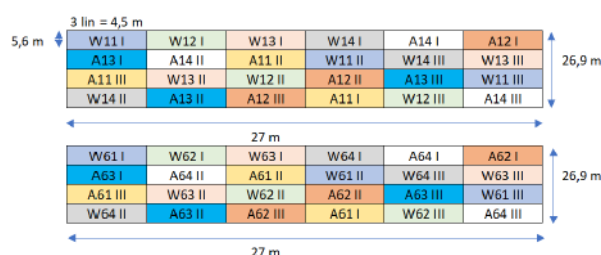
Figura 1.- Esquema de las parcelas para el ensayo de fertilización y riego. Cada parcela es de 5,6 \times 4,5 = 25,2 \text{ m}^2 y las filas estarán separadas por pasillos de 1,5 m
