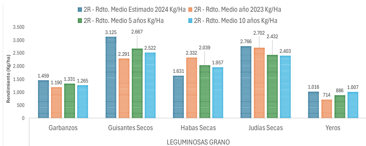
Gráfico 6. Serie histórica de rendimientos en leguminosas grano de regadío (Kg/ha).
