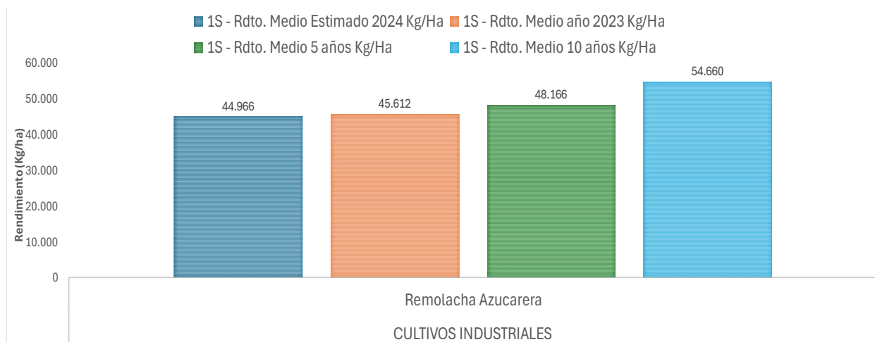
Gráfico 7.2. Serie histórica de rendimientos de remolacha azucarera en secano (Kg/ha).
