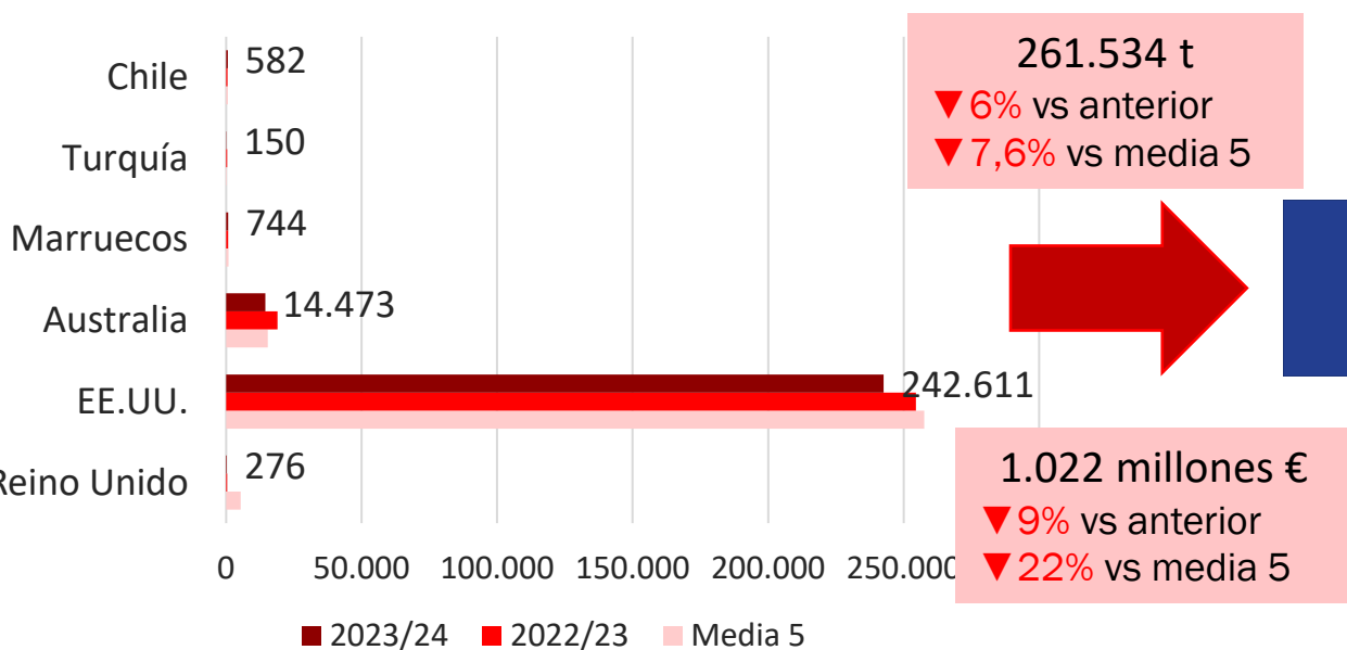
Principales orígenes de importación de almendra por la UE27 - Volumen (t)
